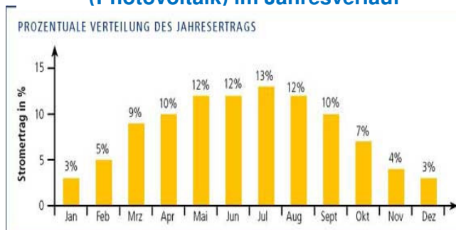
Ertrag einer Solarstromanlage (Photovoltaik) im Jahresverlauf
